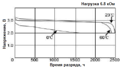
Разряд при различных температурах
