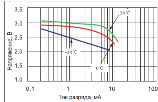
Зависимость напряжения от тока разряда
