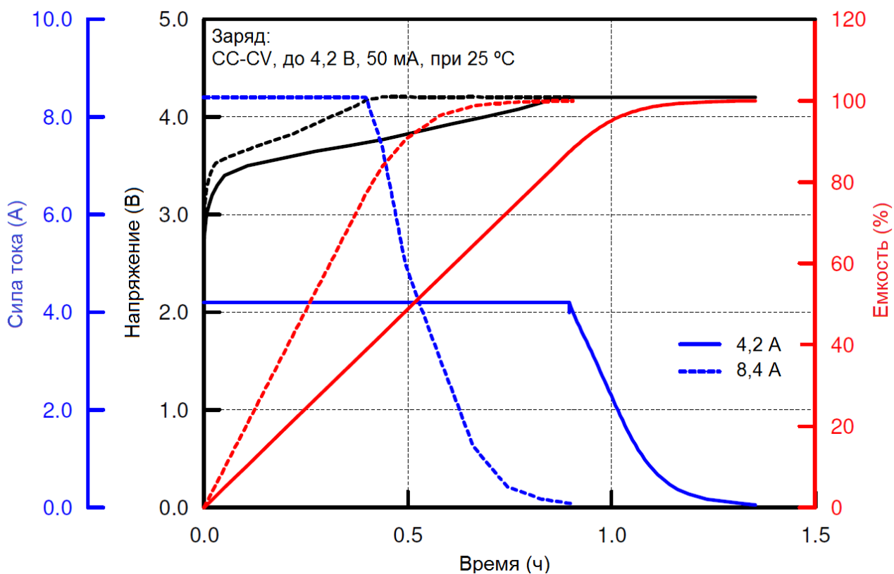
График зависимости емкости, при разных токах разряда.
